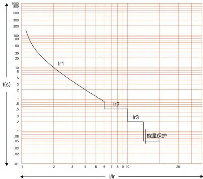
图 5-1 脱扣曲线
